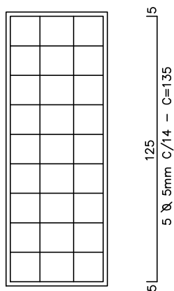
PLANTA
