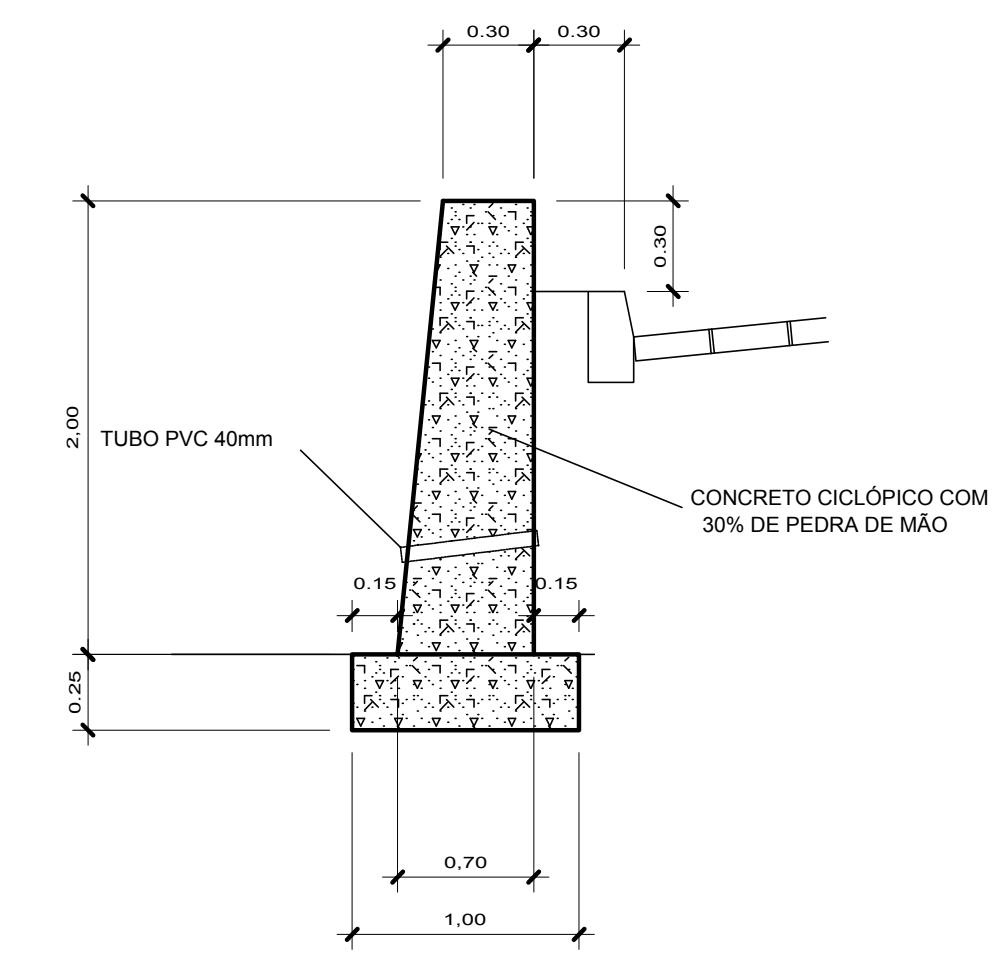
DETALHE DO MURO DE ARRIMO
