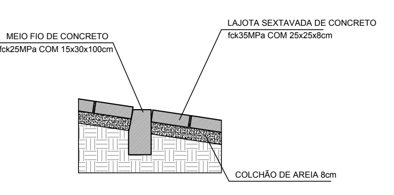
DETALHE DO CINTAMENTO TRANSVERSAL
